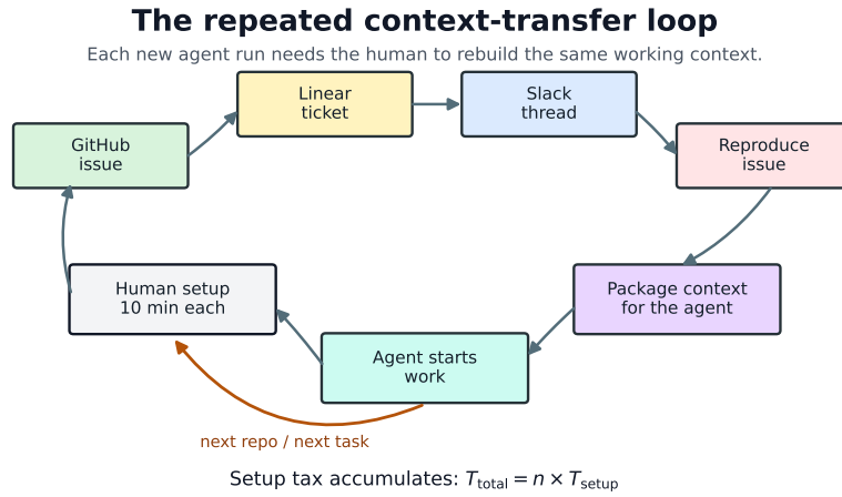
图 2: 上下文转移循环: 每次启动一个智能体, 人都要重新汇集 GitHub issue、Linear ticket、Slack thread 与复现信息, 再把这些隐含状态打包给智能体。若一次启动成本为 T_{\text{setup}} , 重复 n 次后的总成本可写成 T_{\text{total}} = n \times T_{\text{setup}} 。 4
